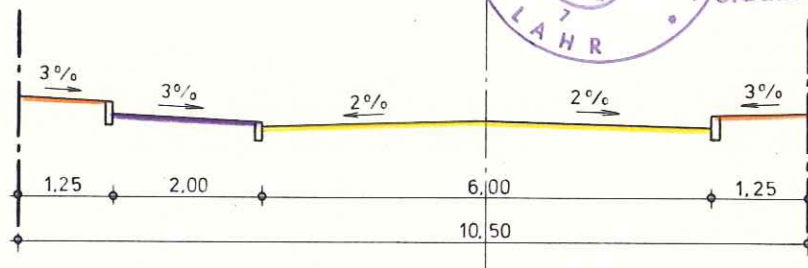
Profil A mit Parkstreifen
