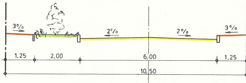
Profil A mit Grünstreifen
